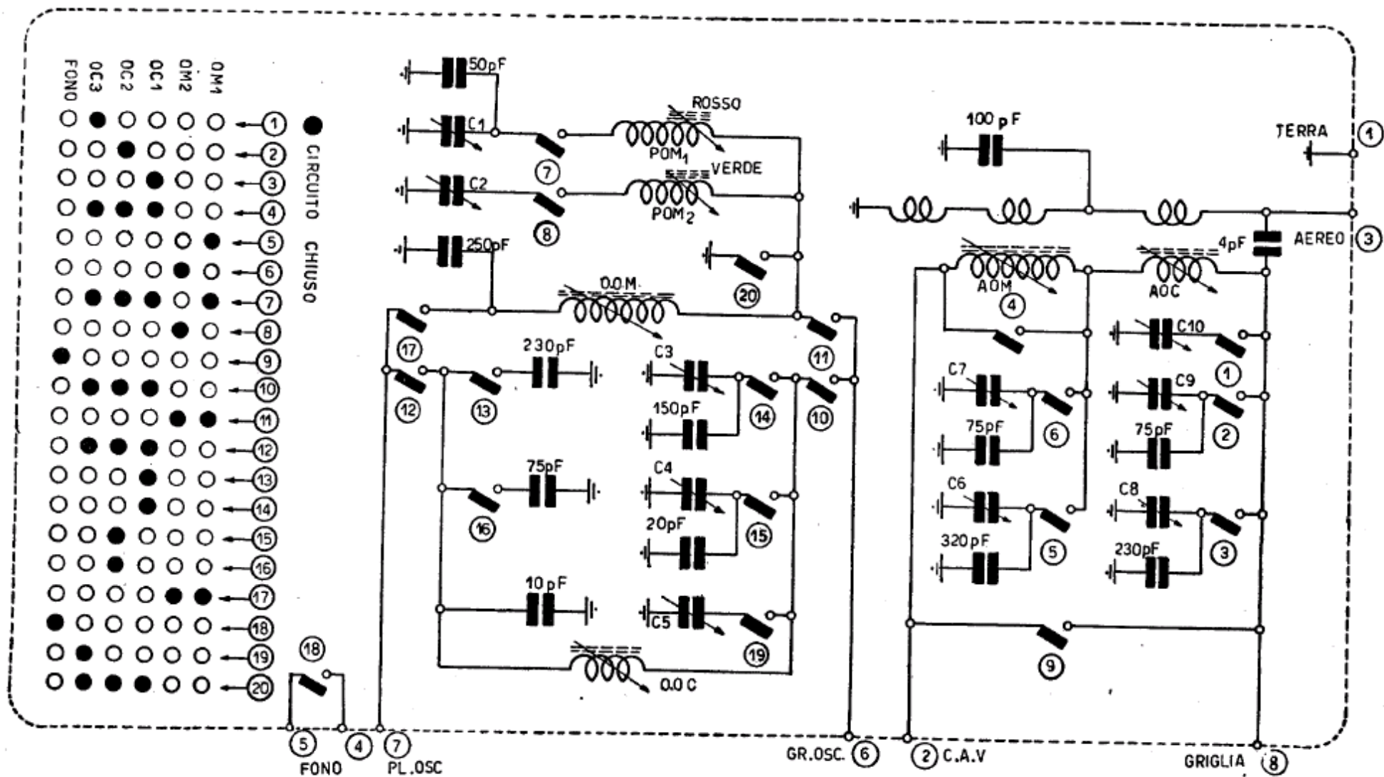
NOVA RADIO - GRUPPO ALTA FREQUENZA Mod P1 - Ad induttori variabili. Gamma onde medie divisa. Tre gamme OC. È presente in alcuni ricevitori, per es. Voce del Padrone 406, Unda R 55/1, ecc.
